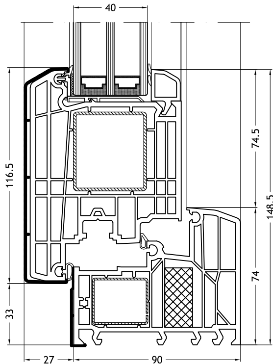
Telaio forma ad L A9240K con anta Step-line Door out
