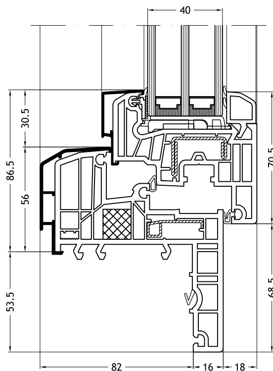
Telaio a Z 129K con anta Step-line C
