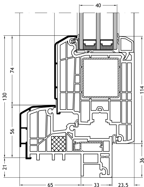
Telaio a Z 923K con anta Step-line Door
