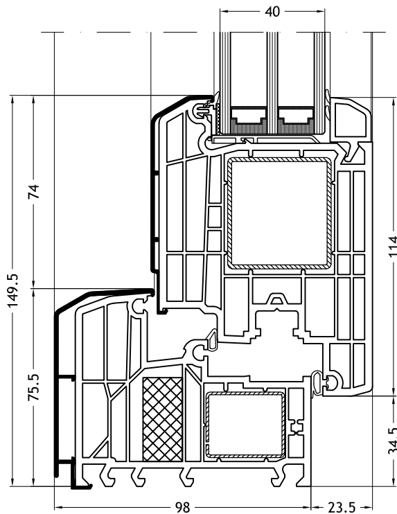
Telaio a L 924K con anta Step-line Door
