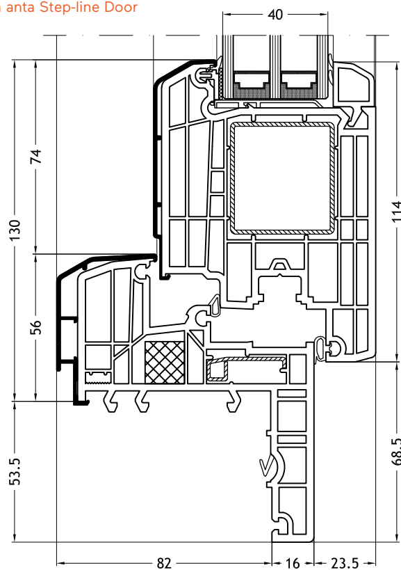
Telaio a Z 129K con anta Step-line Door
