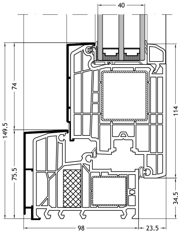
Blendrahmen L-Form 924N mit Flügel Step-line Door
