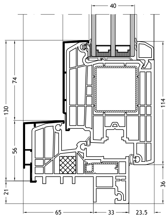
Blendrahmen Z-Form 923N mit Flügel Step-line Door
