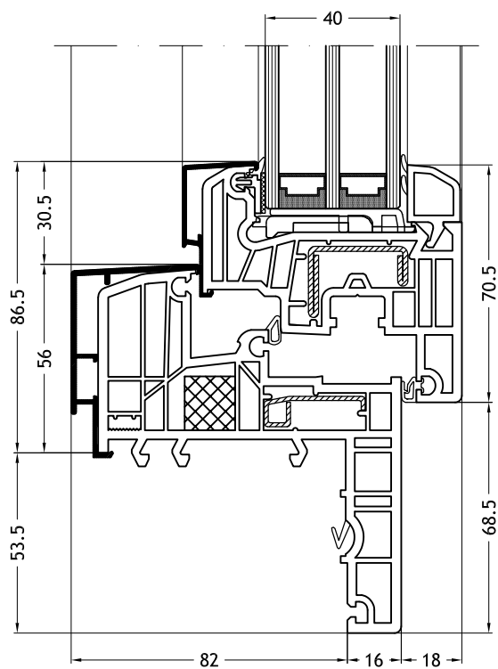
Blendrahmen Z-Form 129N mit Flügel Step-line N
