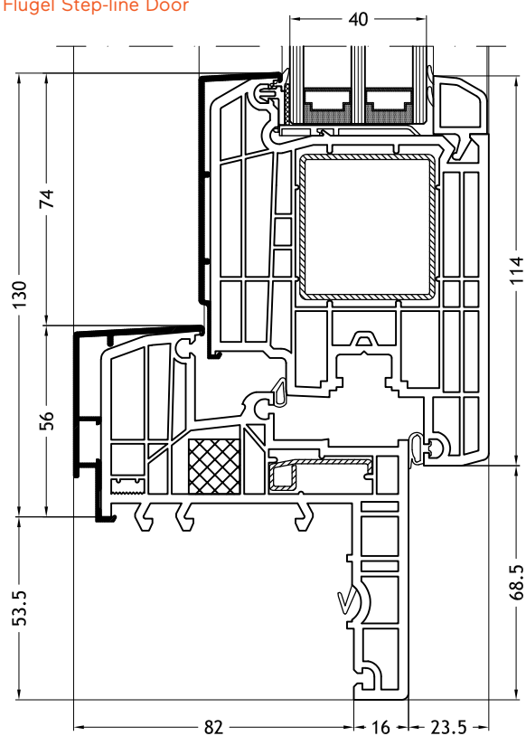
Blendrahmen Z-Form 129N mit Flügel Step-line Door
