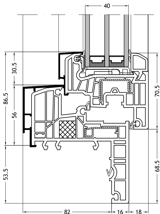
Telaio a Z 129N
