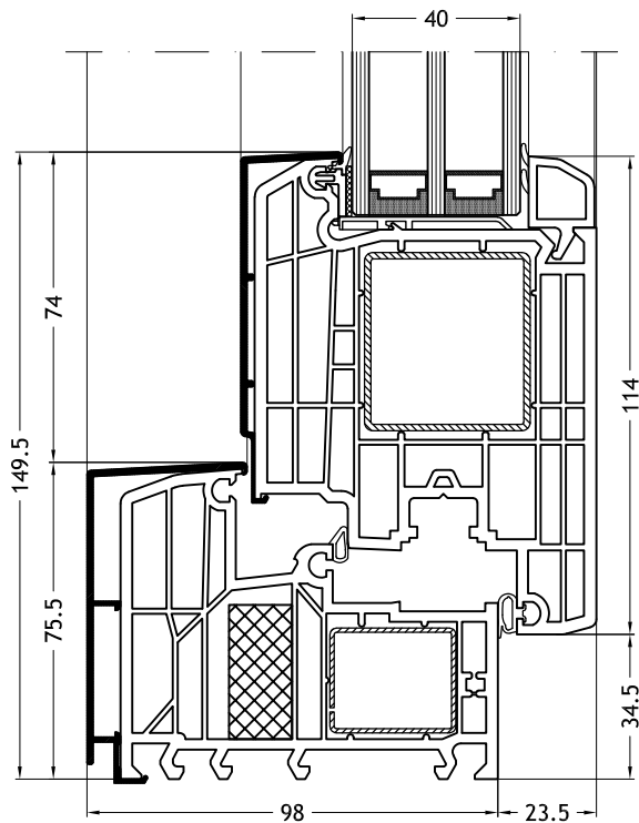
Telaio a L 924N con anta Step-line Door
