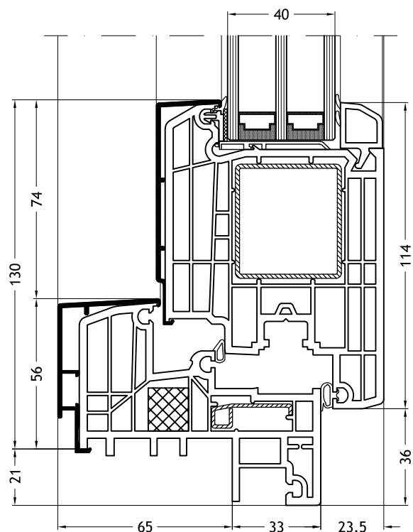
Telaio a Z 923N
