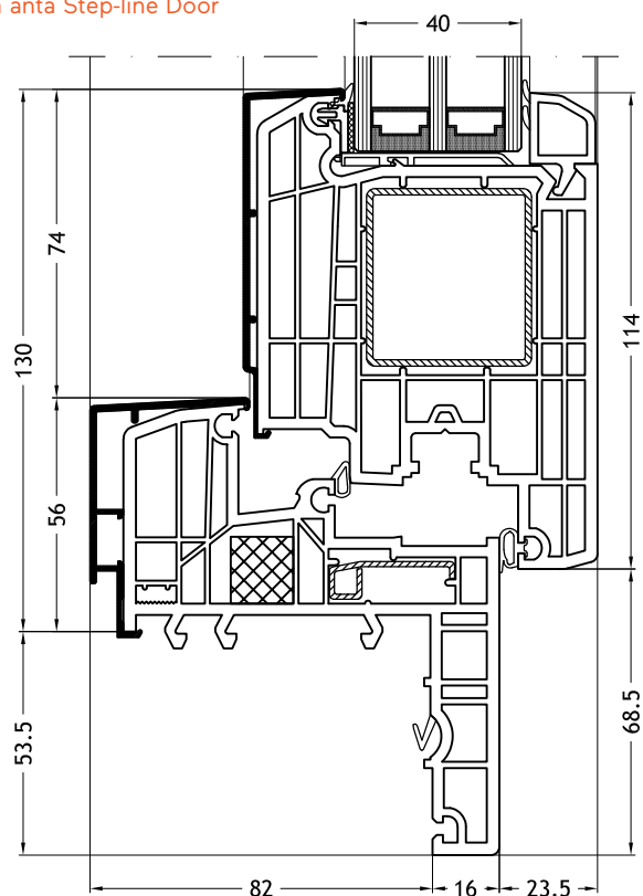
Telaio a Z 129N
