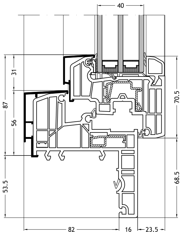
Blindraam Z-vorm 929N met vleugel Step-line N
