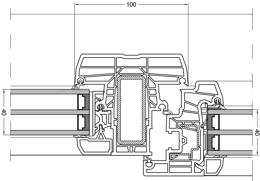
Travessa/montante 922 com folha Classic-line com elemento fixo
