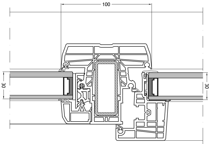
Travessa/montante 922 com folha Nova-line 971 com elemento fixo
