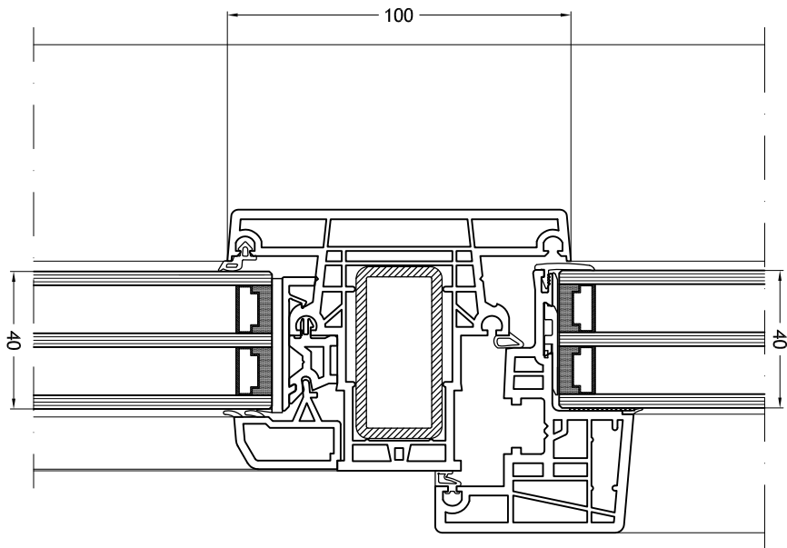
Travessa/montante 969 com folha Nova-line 953 com elemento fixo
