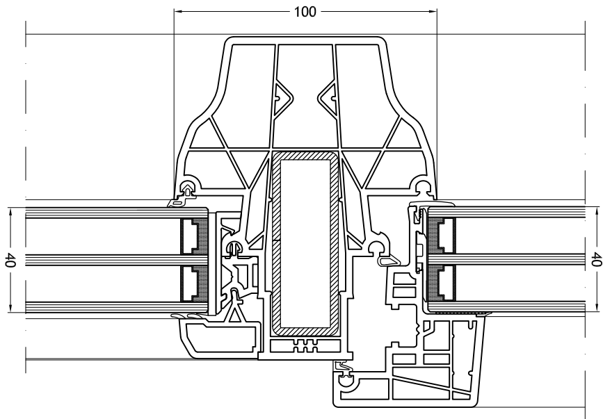
Travessa/montante 952 com folha Nova-line 953 com elemento fixo
