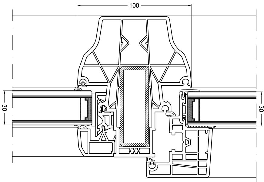
Travessa/montante 952 com folha Nova-line 971 com elemento fixo
