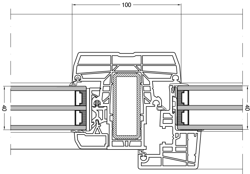
Travessa/montante 922 com folha Nova-line 953 com elemento fixo
