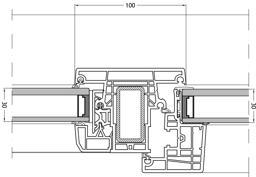
Travessa/montante 969 com folha Nova-line 971 com elemento fixo
