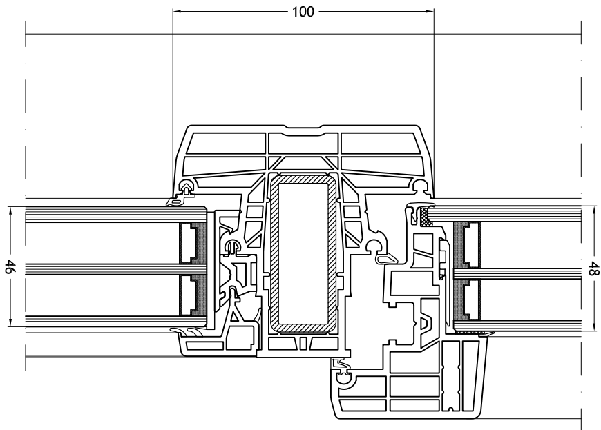
Travessa/montante 922 com folha Nova-line Plus com elemento fixo
