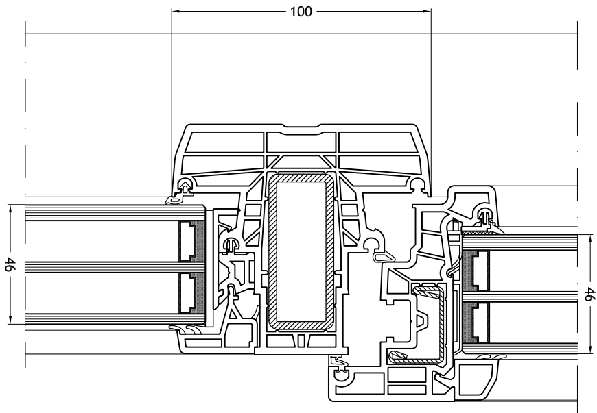
Travessa/montante 922 com folha Slim-line com elemento fixo
