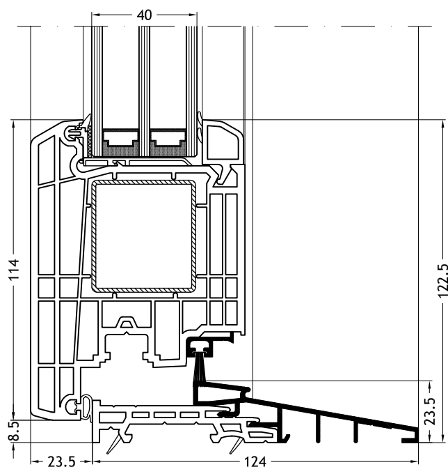
Seuil plat avec ouvrant Step-line Door out
