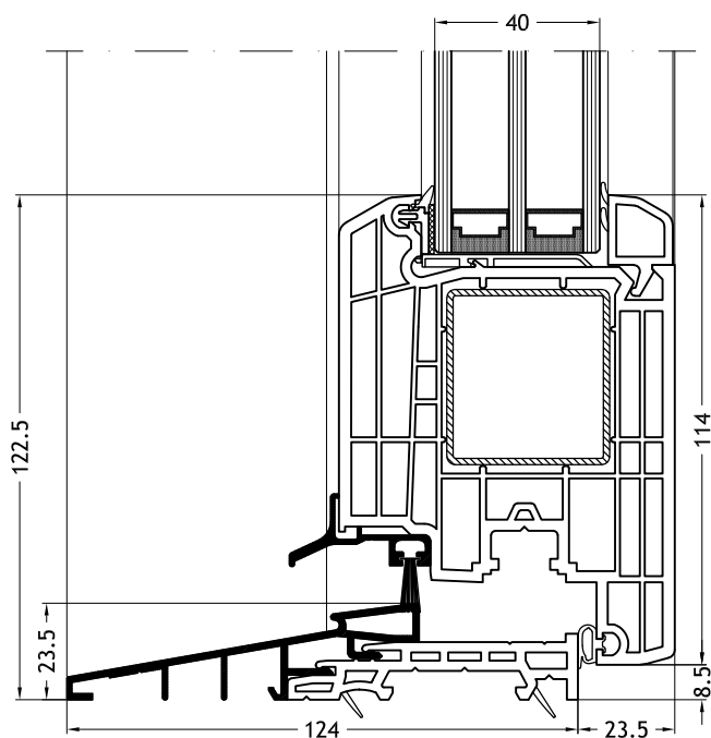
Seuil plat avec ouvrant Step-line Door
