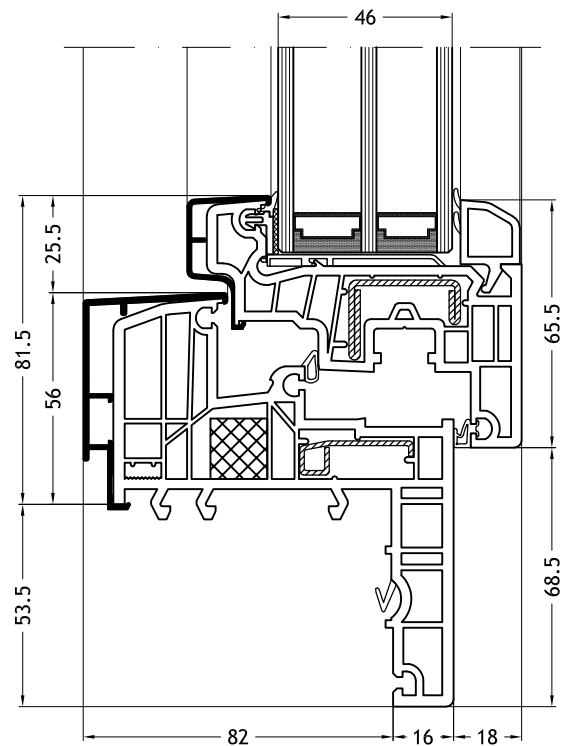
Telaio a Z 129N con anta Slim-line N
