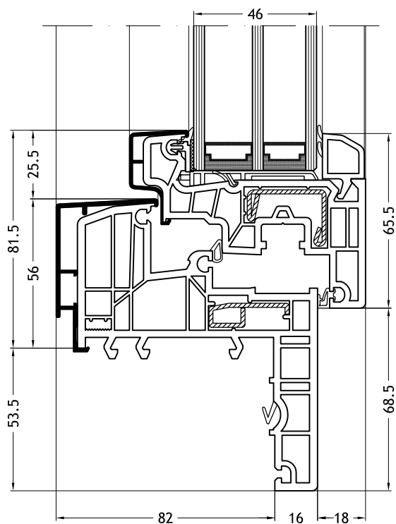
Dormant en L, 929N avec ouvrant Slim-line N
