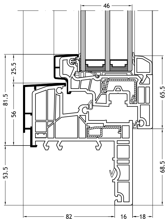
Blindraam L-vorm 929N met vleugel Slim-line N
