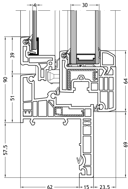
Blendrahmen Z-Form 966 mit Flügel Slim-line Twin
