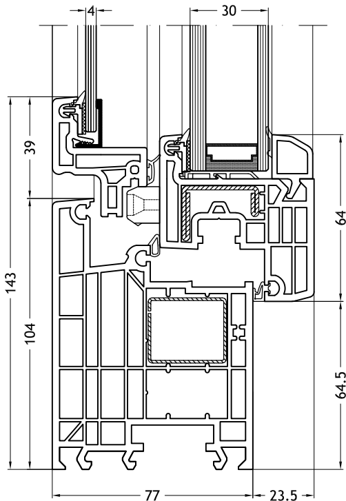
Blendrahmen L-Form 963 mit Flügel Slim-line Twin
