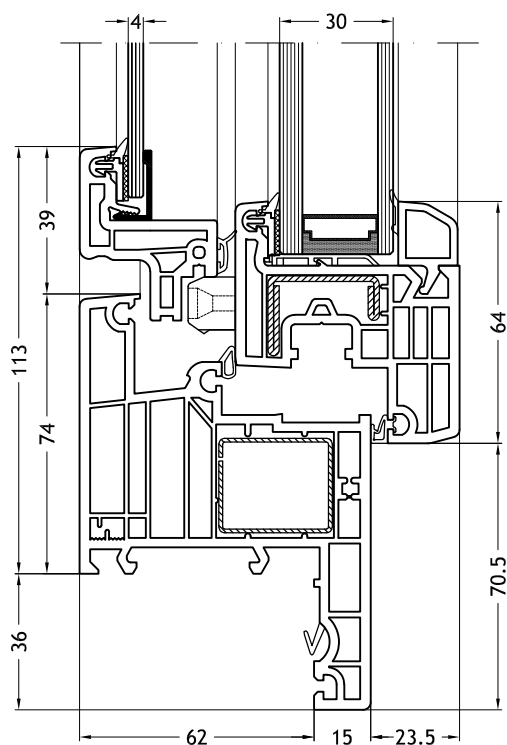
Blendrahmen Z-Form 967 mit Flügel Slim-line Twin
