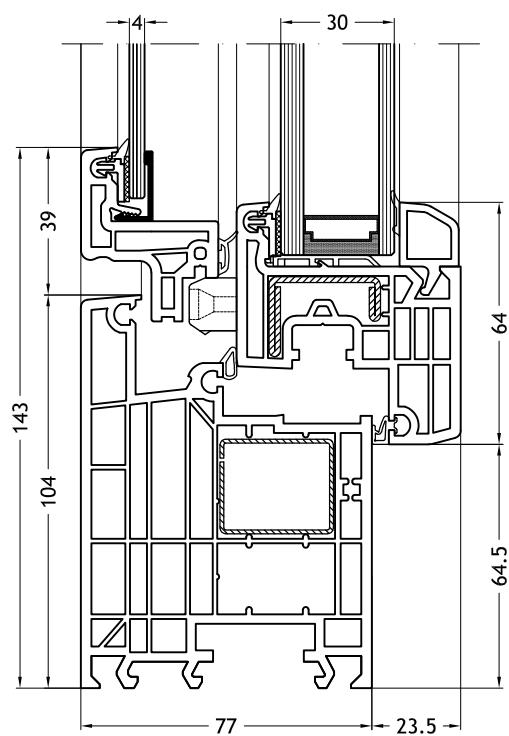
Telaio a L 963 con anta Slim-line Twin
