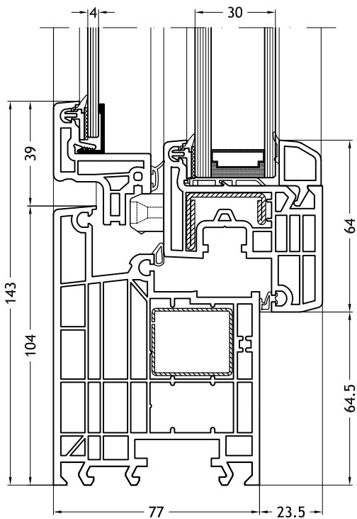
Marco L, 963 con hoja Slim-line Twin
