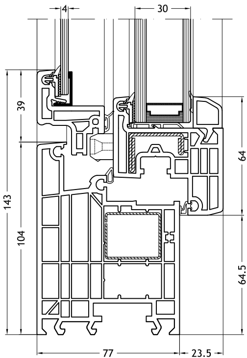
Kozijn L-vorm 963 met vleugel Slim-line Twin
