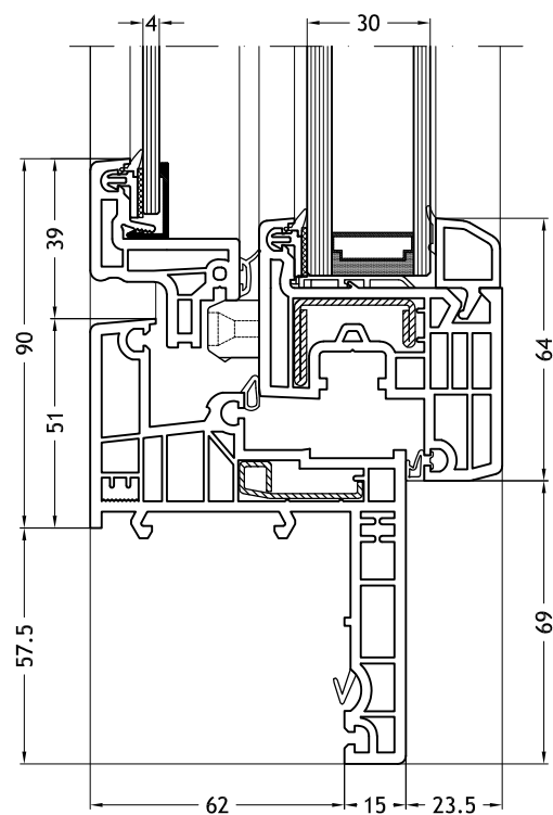
Kozijn Z-vorm 966 met vleugel Slim-line Twin
