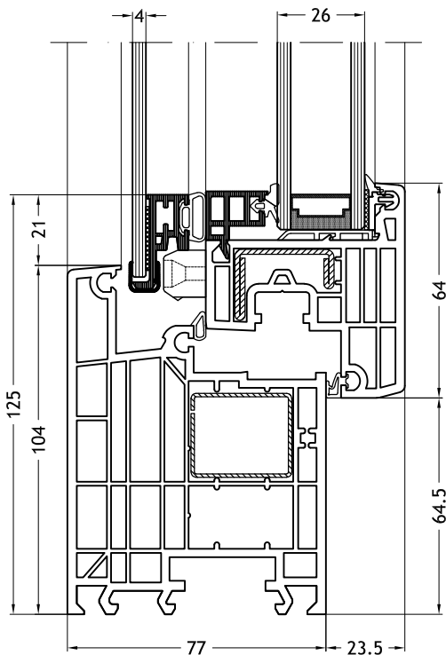
Blendrahmen L-Form 963 mit Flügel Nova-line Twin
