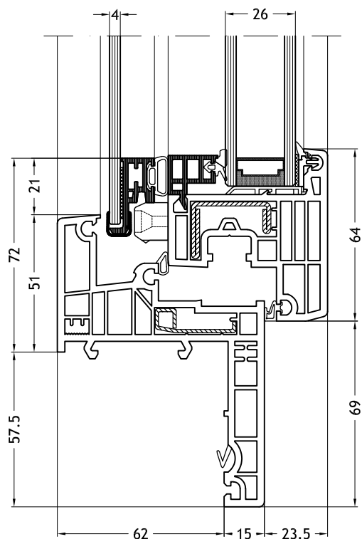
Blendrahmen Z-Form 966 mit Flügel Nova-line Twin
