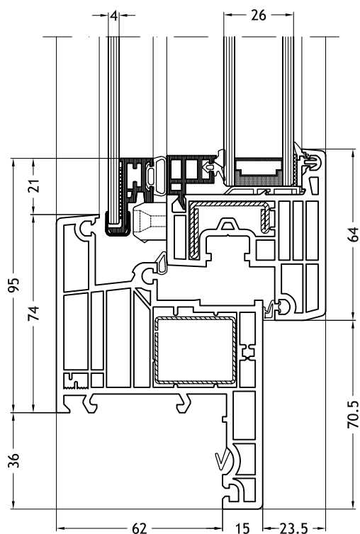
Blendrahmen Z-Form 967 mit Flügel Nova-line Twin
