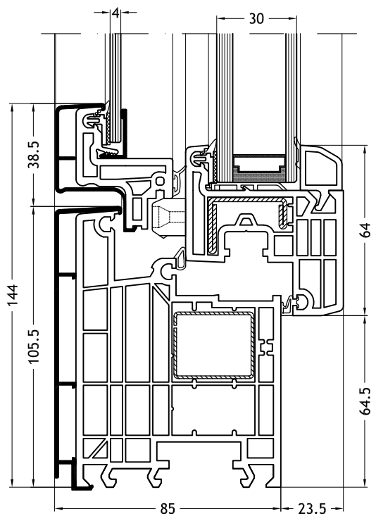
Telaio a L 963N con anta Slim-line Twin
