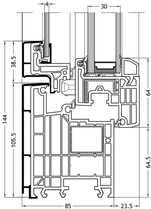
Dormant en L, 963N avec ouvrant Slim-line Twin
