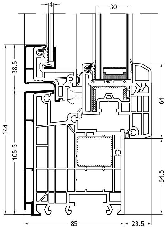
Kozijn L-vorm 963N met vleugel Slim-line Twin
