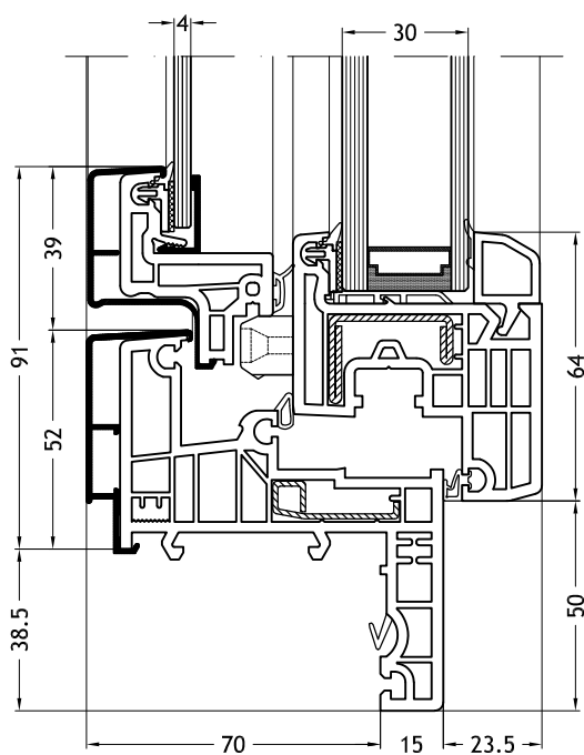
Kozijn Z-vorm 965N met vleugel Slim-line Twin
