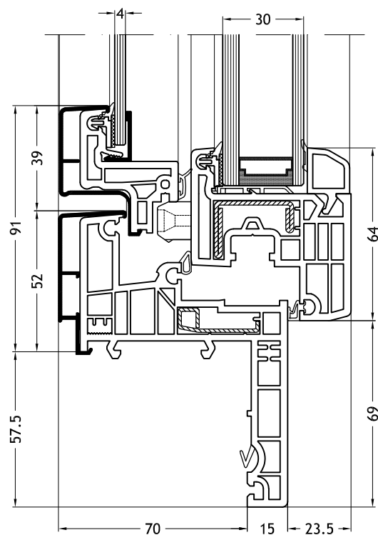
Kozijn Z-vorm 966N met vleugel Slim-line Twin
