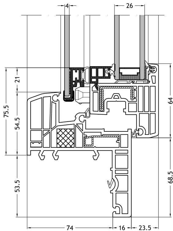
Kozijn Z-vorm 929 met vleugel Nova-line Twin
