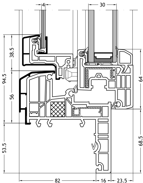
Telaio a Z 129K con anta Slim-line Twin C
