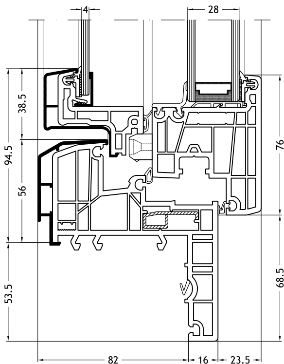
Blindraam Z-vorm 929K met vleugel Slim-line Twin C
