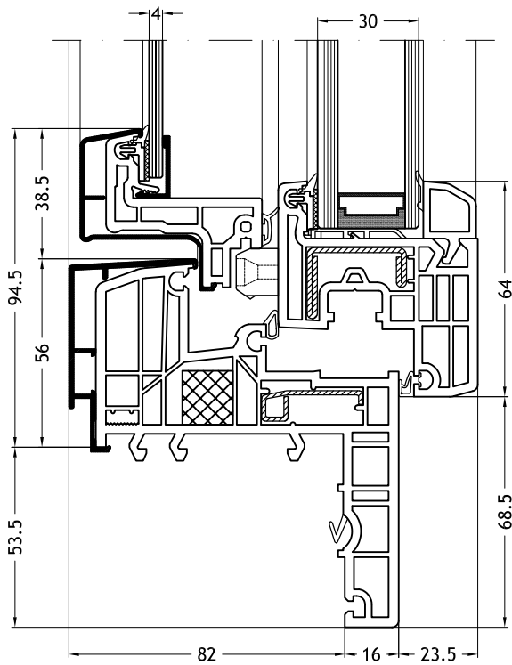
Blendrahmen Z-Form 129N mit Flügel Slim-line Twin N
