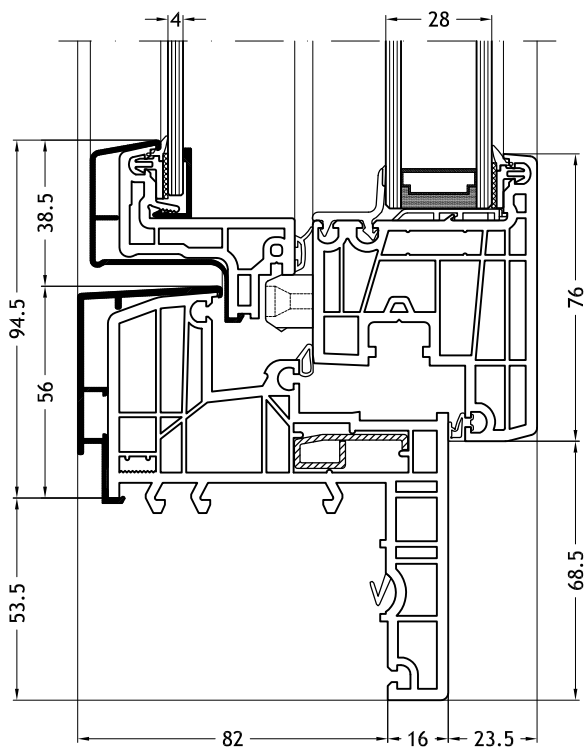
Aro em forma de Z 929N com folha Slim-line Twin N
