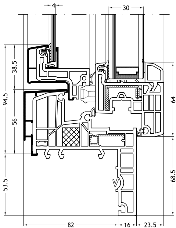
Telaio a Z 129N con anta Slim-line Twin N
