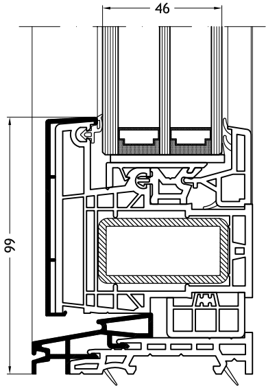
Vlakke onderdorpel met vast raam
