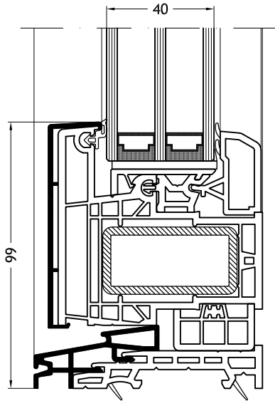
Vlakke onderdorpel met vast raam
