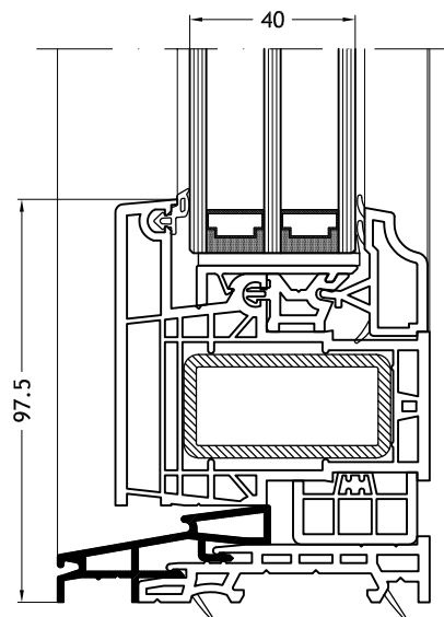
Soleira plana com elemento fixo com bite estilo
