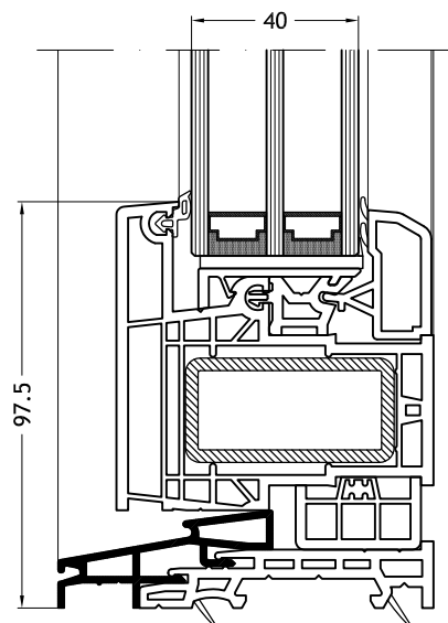
Soleira plana com elemento fixo
