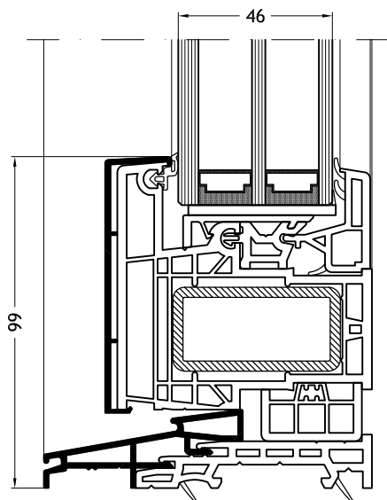
Soleira plana com elemento fixo C
