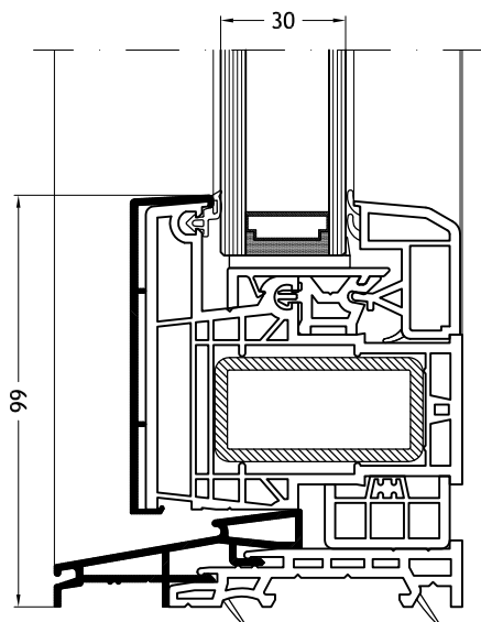
Vlakke onderdorpel met vast raam C
