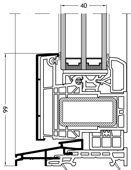
Vlakke onderdorpel met vast raam C
