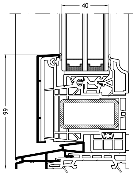
Vlakke onderdorpel met vast raam C met glaslat stijl
