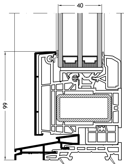
Soleira plana com elemento fixo
