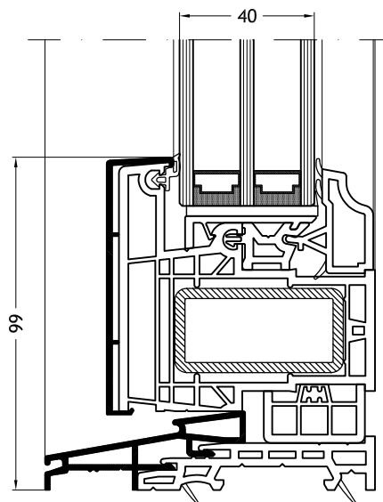
Soleira plana com elemento fixo N com bite estilo
