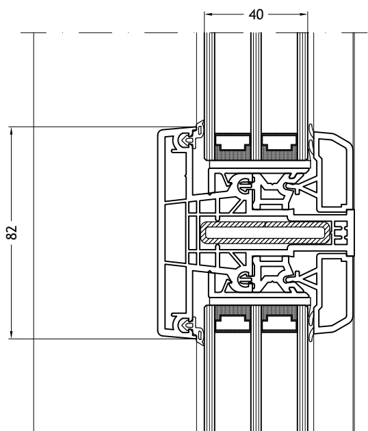
Montant/traverse 968 avec et châssis fixe
