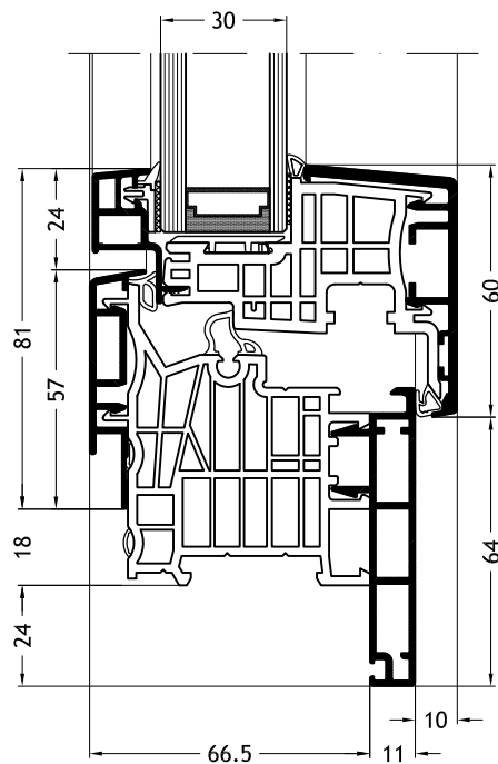
Dormant en L, D1Y avec ouvrant Slim-line A16
