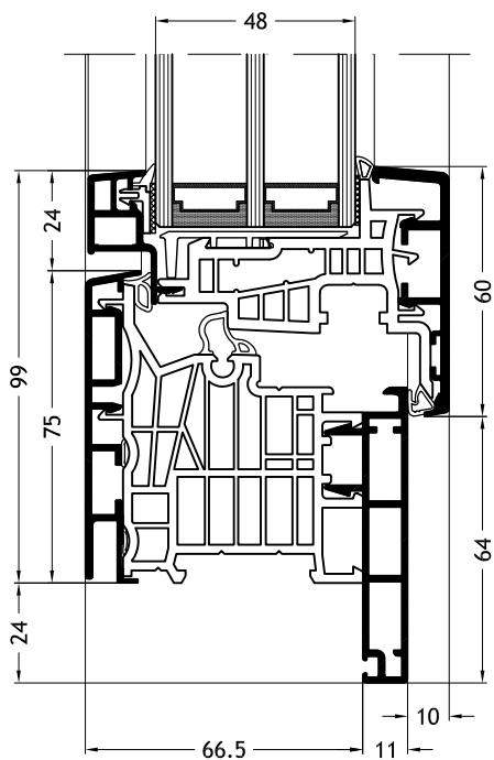
Dormant en L, D1W avec ouvrant Slim-line A17
