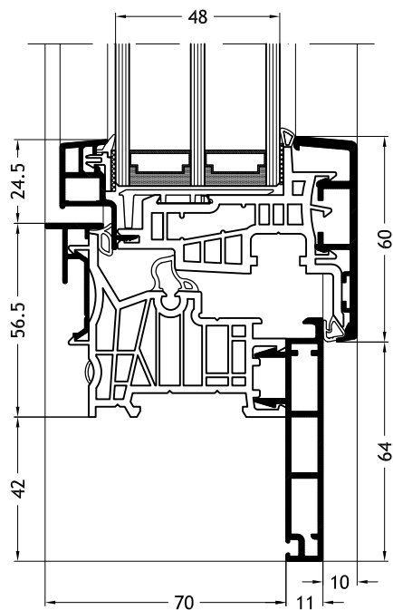
Dormant en Z, D2X avec ouvrant Slim-line A17
