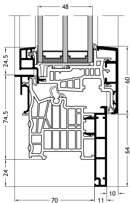
Dormant en L, D1X avec ouvrant Slim-line A17
