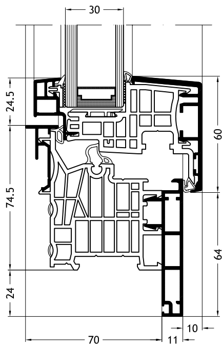
Dormant en L, D1X avec ouvrant Slim-line A16
