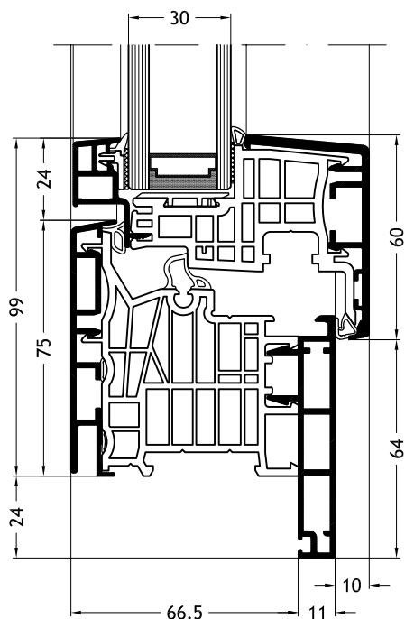
Dormant en L, D1W avec ouvrant Slim-line A16
